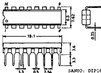
外形図 3064-D16TR (unit: mm)
