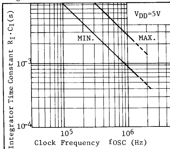
Fig.10 R_I \cdot C_I - f_{OSC}
