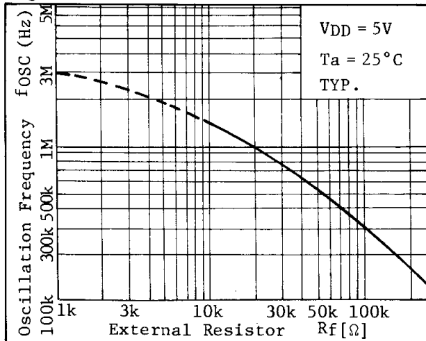
Fig. 5 R_f - f_{OSC}
