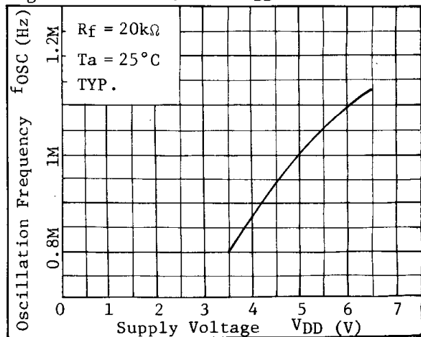
Fig. 6 f_{OSC} - V_{DD}
