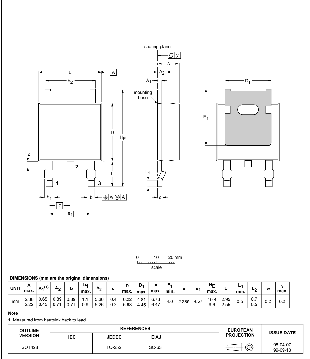
Fig 16. SOT428 (D-PAK).
