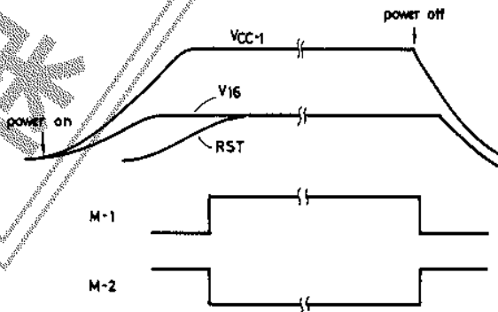
図3 電源 オン、オフ 時のミュート動作
