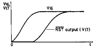
図2 電源オン時のリセット出力
