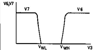
図1 同期検出回路入出力特性
