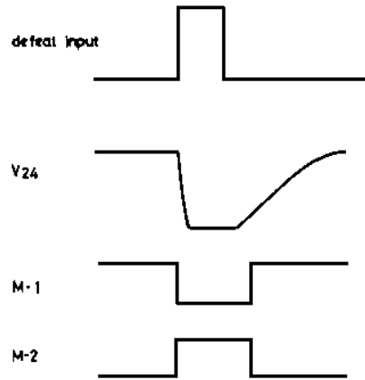
図4 デフィート入力時のミュート動作
