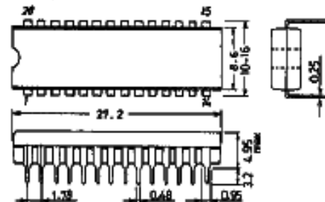
外形図 3029A-D28SIC (unit: mm)
