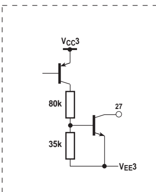
Fig. 8e Lock detect output
