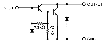
TD62101P/F
