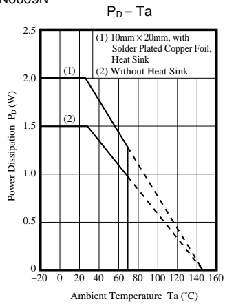
AN6608, AN6609N
