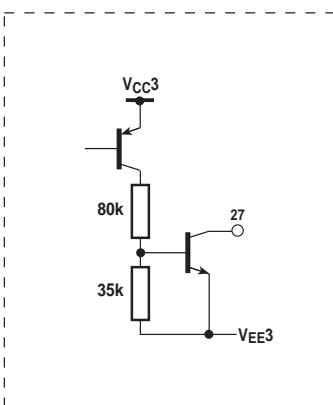
Fig. 8e Lock detect output
