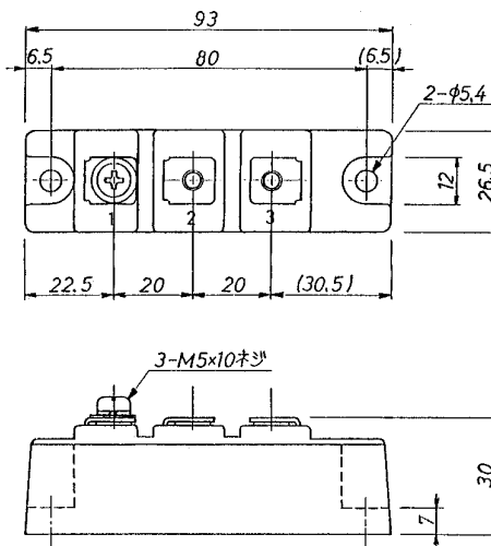
外形寸法図 OUTLINE DRAWING (単位 Dimension : mm)
