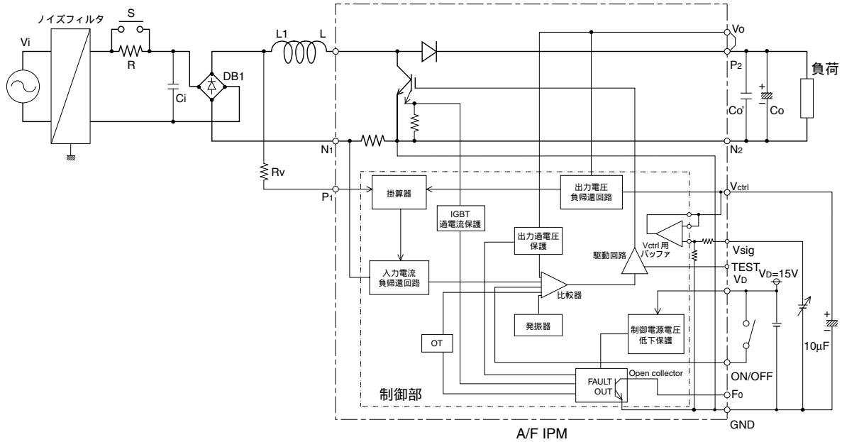
図2. PM52AUBZ060-1 内部機能ブロック図
