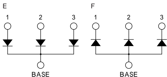
回路図 CIRCUIT
