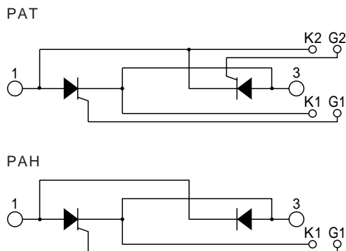
回路図 CIRCUIT
