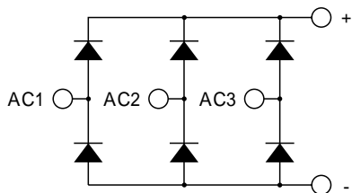
回路図 CIRCUIT
