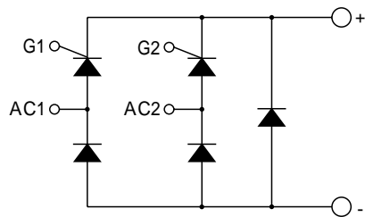
回路図 CIRCUIT
