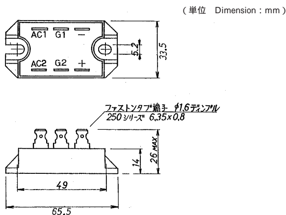
外形寸法図 OUTLINE DRAWING
