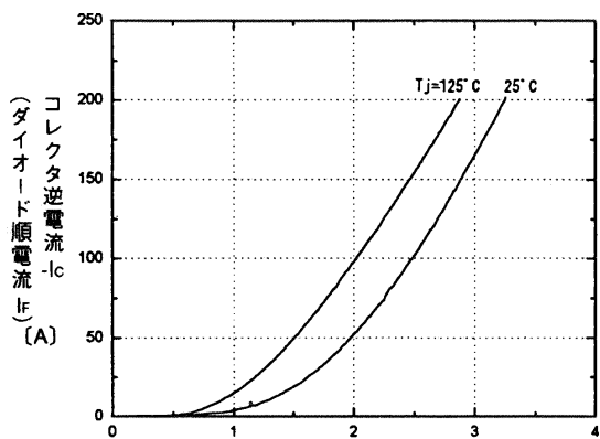
コレクタ逆電流 -I_c (ダイオード順電流 I_F ) (A) T_j=125^\circ\text{C} 25^\circ\text{C} エミッタ・コレクタ間電圧 V_{ceD} (V) (ダイオード順電圧 V_F ) 高速フリーホイールダイオード順電圧特性 <INV部> Forward voltage of free wheel diode <INV>
