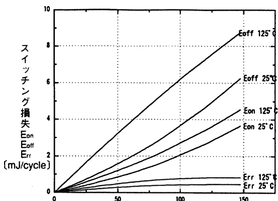
スイッチング損失 E_{on} , E_{off} , E_{err} (mJ/cycle) E_{on} E_{off} E_{err} T_j=125^\circ\text{C} 25^\circ\text{C} コレクタ電流 I_c (A) スイッチング損失-コレクタ電流特性 <INV部> Switching loss vs. Collector current <INV>
