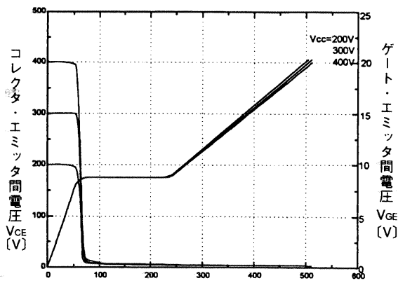
コレクタ・エミッタ間電圧 V_{ce} (V) ゲート・エミッタ間電圧 V_{ge} (V) 充電電荷量 Q_g (nC) ダイナミック入力特性 ( T_j=25^\circ\text{C} ) <INV部> Dynamic input characteristic <INV>
