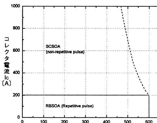
コレクタ電流 I_c (A) コレクタ・エミッタ間電圧 V_{ce} (V) SCSOA (non-repetitive pulse) RBSOA (Repetitive pulse) 安全動作領域(逆バイアス) ( T_j \leq 125^\circ\text{C} ) <INV部> Reverse biased safe operating area <INV>
