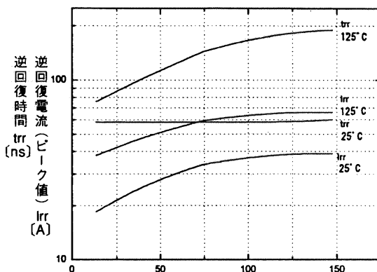
逆回復時間 t_{rr} (ns) 逆回復電流 (ピーク値) I_{rr} (A) t_{rr} I_{rr} 特性 <INV部> t_{rr} , I_{rr} <INV>
