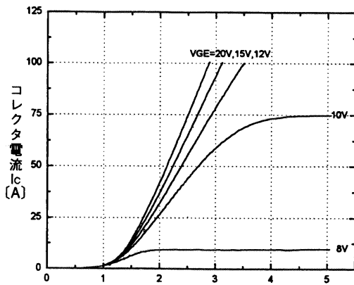
コレクタ電流-コレクタ・エミッタ間電圧特性(Tj=25°C)<ブレーキ部> Collector current vs. Collector-Emitter voltage<BRAKE>
