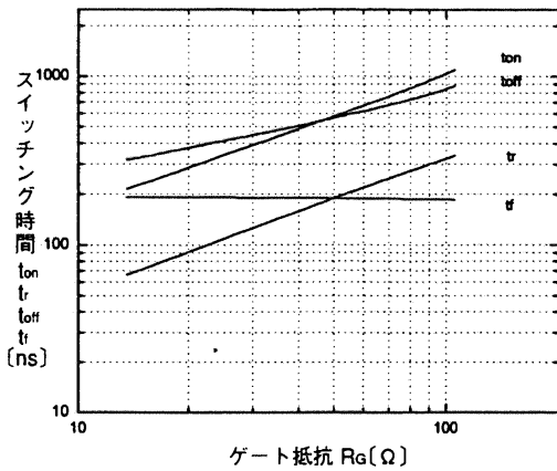
スイッチング時間-ゲート抵抗特性 ( T_j=25^\circ\text{C} ) <ブレーキ部> Switching time vs. Gate resistance <BRAKE>
