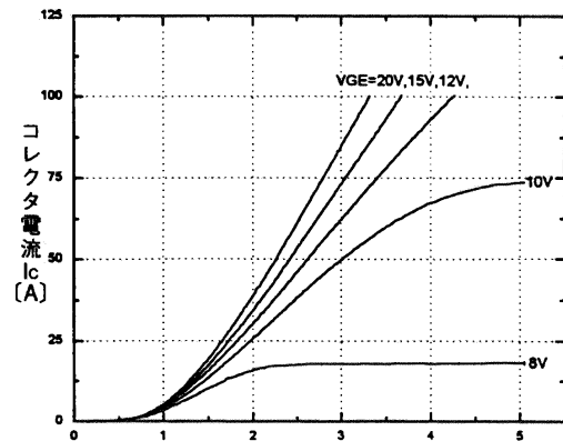
コレクタ電流-コレクタ・エミッタ間電圧特性(Tj=125°C)<ブレーキ部> Collector current vs. Collector-Emitter voltage<BRAKE>
