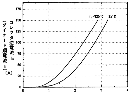
エミッタ・コレクタ間電圧 V_{ce} (V) (ダイオード順電圧 V_F ) 高速フリーホイールダイオード順電圧特性 <INV部> Forward voltage of free wheel diode <INV>
