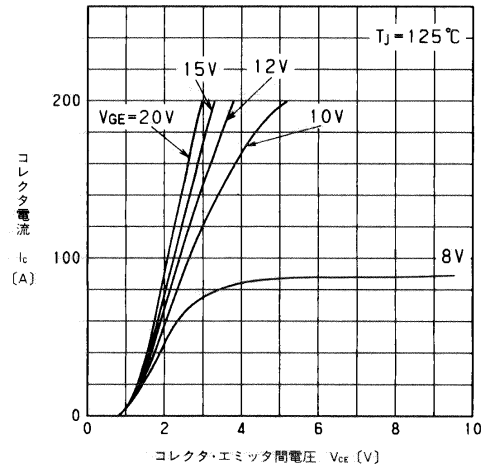
コレクタ電流—コレクタ・エミッタ間電圧特性 Collector Current vs. Collector-Emittor Voltage
