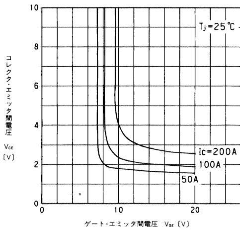
コレクタ・エミッタ間電圧—ゲート・エミッタ間電圧特性 Collector-Emittor Voltage vs. Gate-Emittor Voltage
