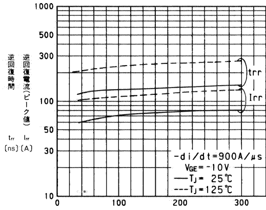
T_{rr} , I_{rr} - I_F 特性 T_{rr} , I_{rr} - I_F
