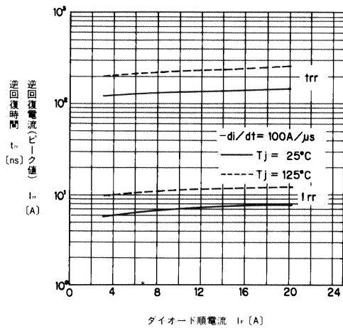
t_{rr} , I_{rr} - I_c 特性 T_{rr} , I_{rr} - I_c
