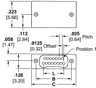
Receptacle
