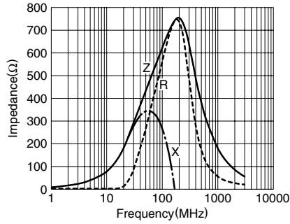
MMZ2012Y202B
