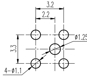
安装孔 PIERCING PLAN
