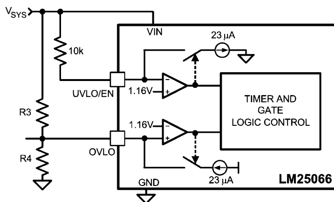
FIGURE 12. UVLO = POR
