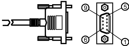
F10-VR2 RS-232C Cable: D-sub 9-pin connector (2 m)
