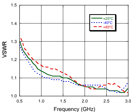
VSWR, 39 pF
