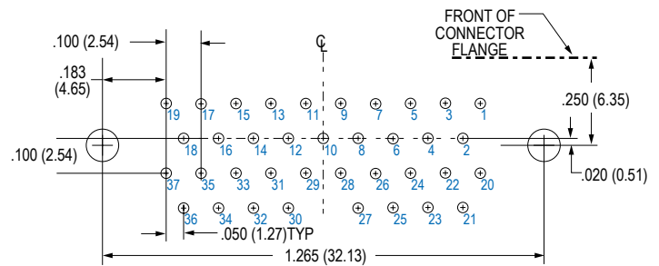
37 SOCKET MWDM-37SCBR
