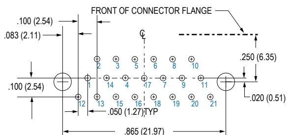
21 PIN MWDM-21PCBR
