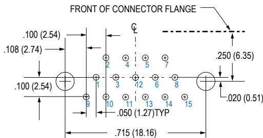
15 PIN MWDM-15PCBR
