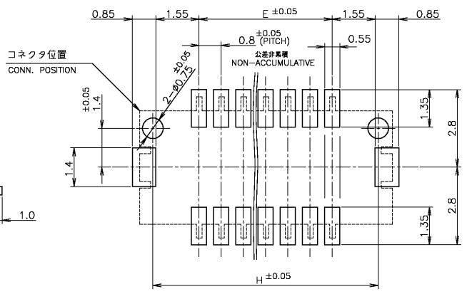
参考基板加工寸法 REFERENCE P.C. BOARD LAYOUT
