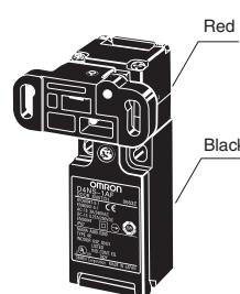
D4NS-1□F + D4DS-K5
