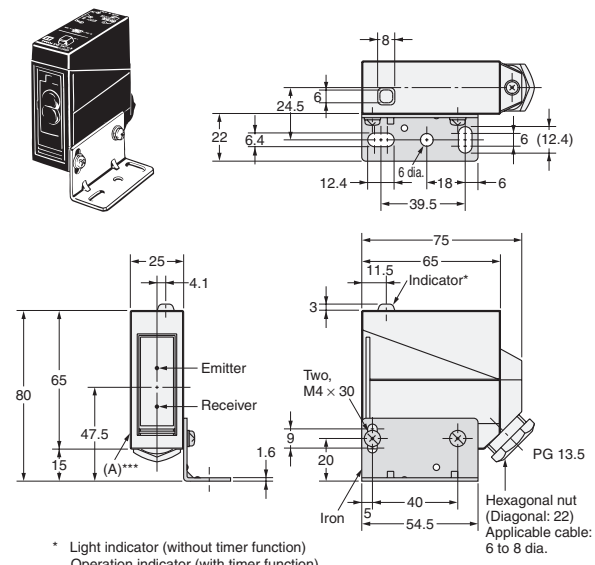
E3JM-DS70□4(T) E3JM-R4□4(T)
