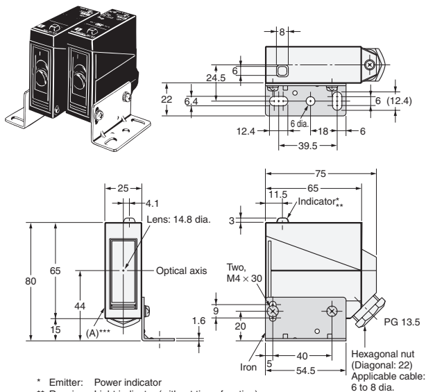
E3JM-10□4T
