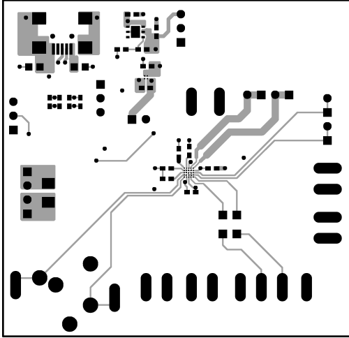
Top Layer
