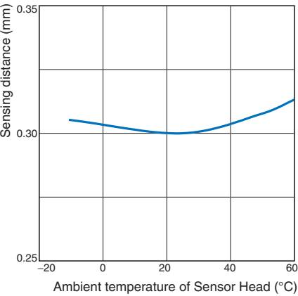
E2C-EM07(-□)
