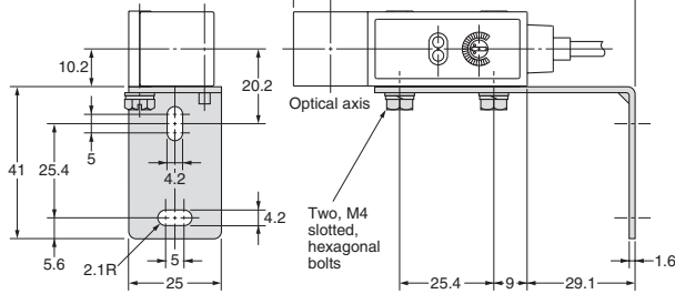
E39-L5
