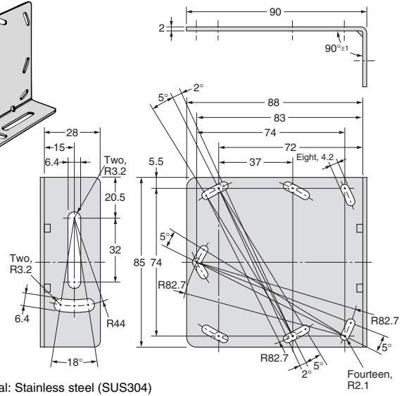
E39-L136
