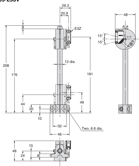
E39-L93V
