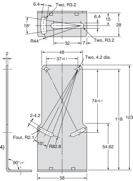
E39-L136
