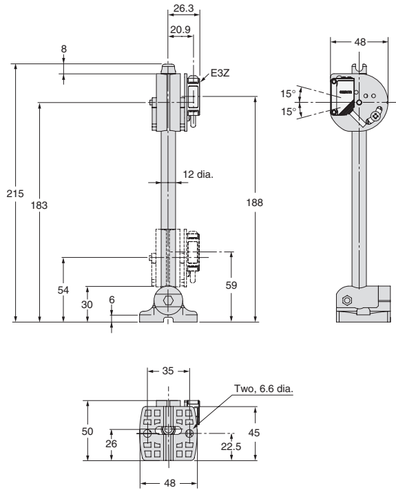
E39-L93H
