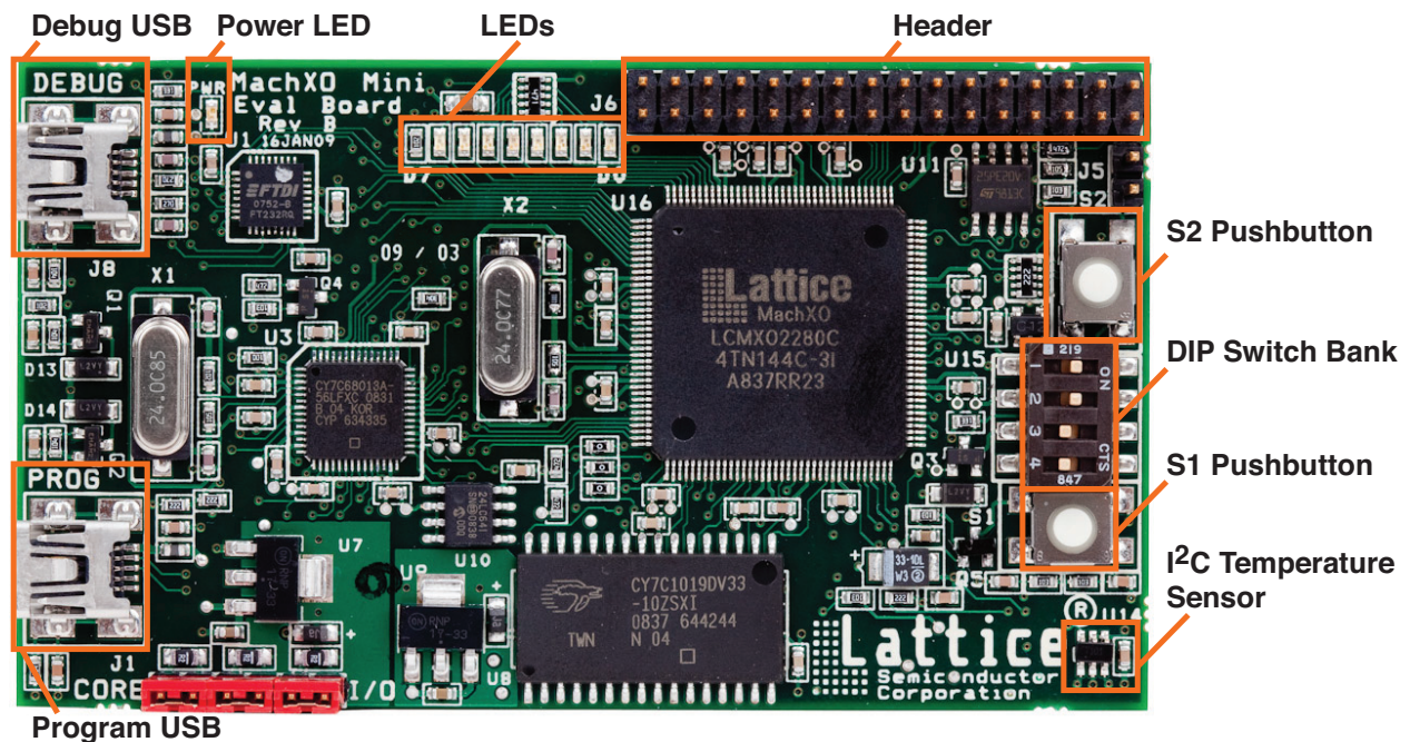
MachXO Mini Evaluation Board Layout Diagram
