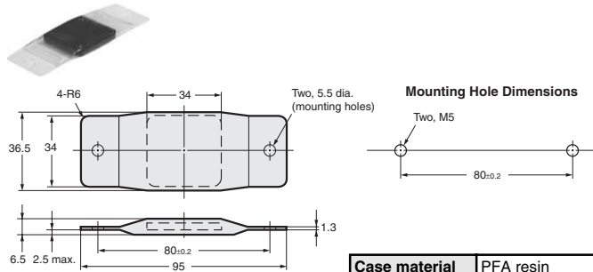
V680-D8KF67/-D8KF67M
