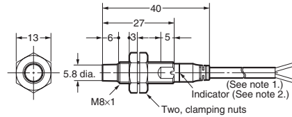
E2A-S08KN04-WP-□□
