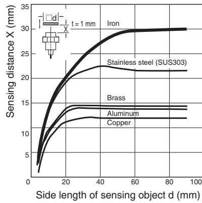
E2A-M30LN30/E2A-S30LN30
