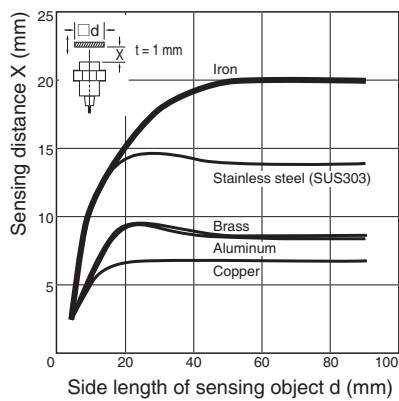
E2A-M30KN20/E2A-S30KN20
