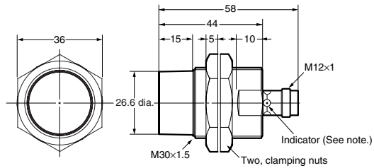
E2A-M30KN20-M1-□□/E2A-S30KN20-M1-□
