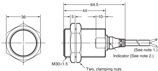
E2A-M30KS15-WP-□□/ E2A-S30KS15-WP-□
