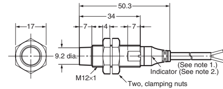
E2A-M12KN08-WP-□□/ E2A-S12KN08-WP-□
