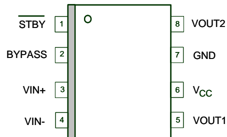
TS4990ID/TS4990IDT - SO-8
