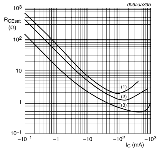
T_{amb} = 25^\circ C (1) I_C/I_B = 100 (2) I_C/I_B = 50 (3) I_C/I_B = 10
