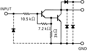
ULN2804APG / AFWG
