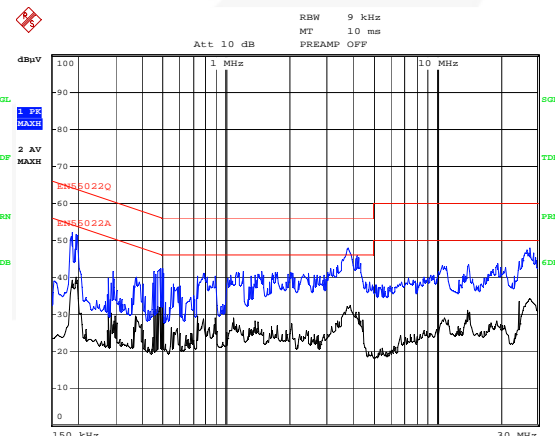
Figure 20. N: 230 / 50Hz
