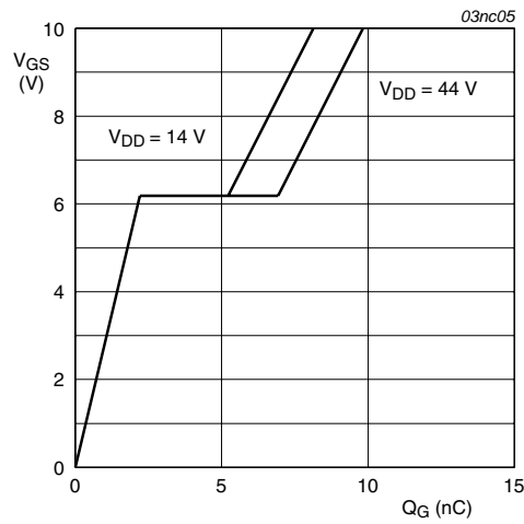
T_j = 25^\circ\text{C}; I_D = 10\text{A}
