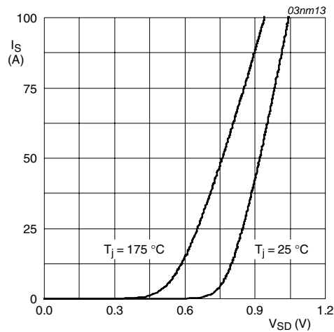
V_{GS} = 0\text{V}
