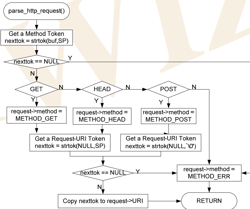
<Fig 3.20: parse_http_request()>
