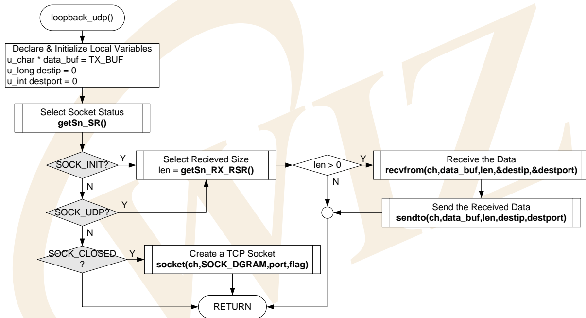
<Fig 3.16: loopback_udp(>
