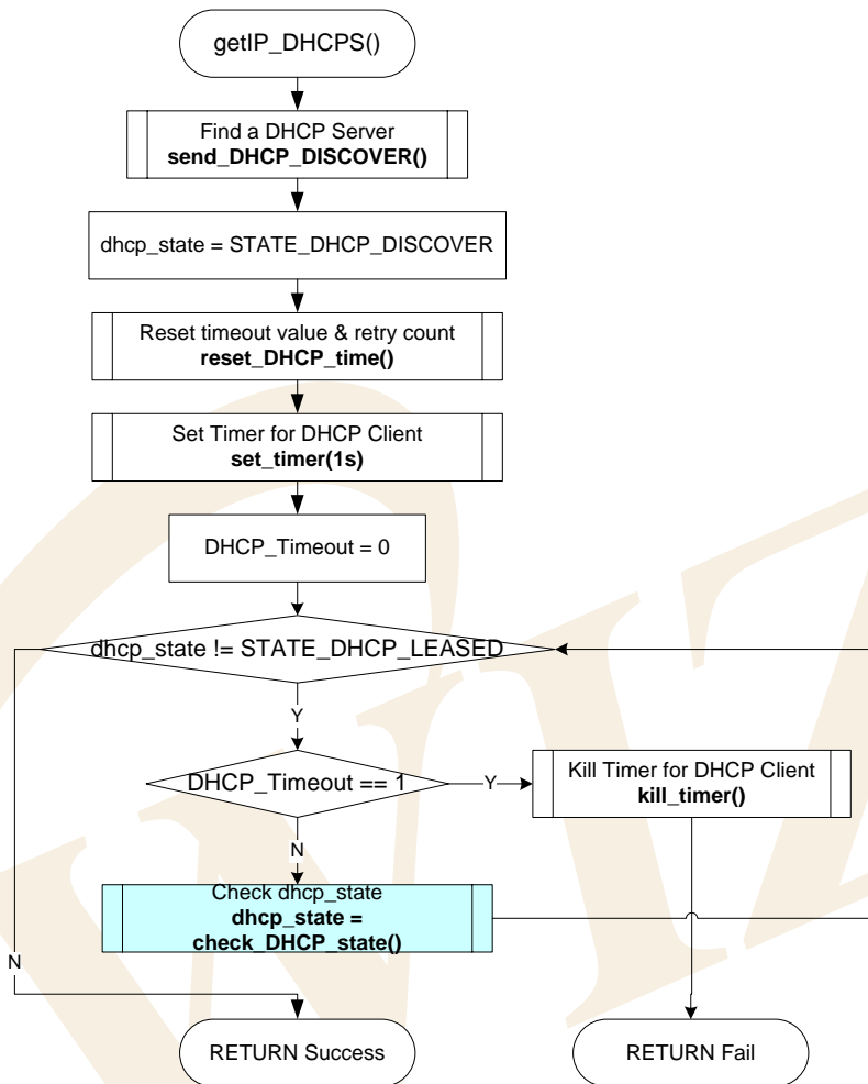
<Fig 3.29: getIP_DHCP()>
