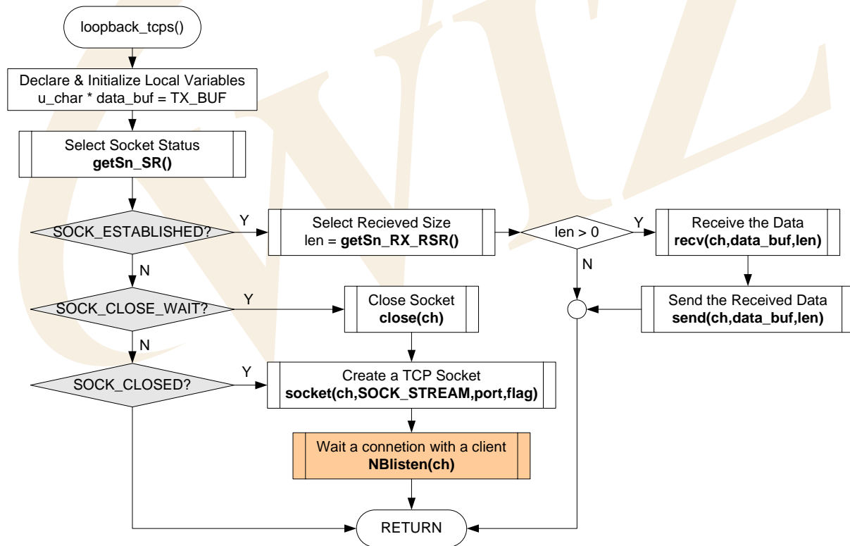
< Fig 3.14 : loopback_tcps() >
