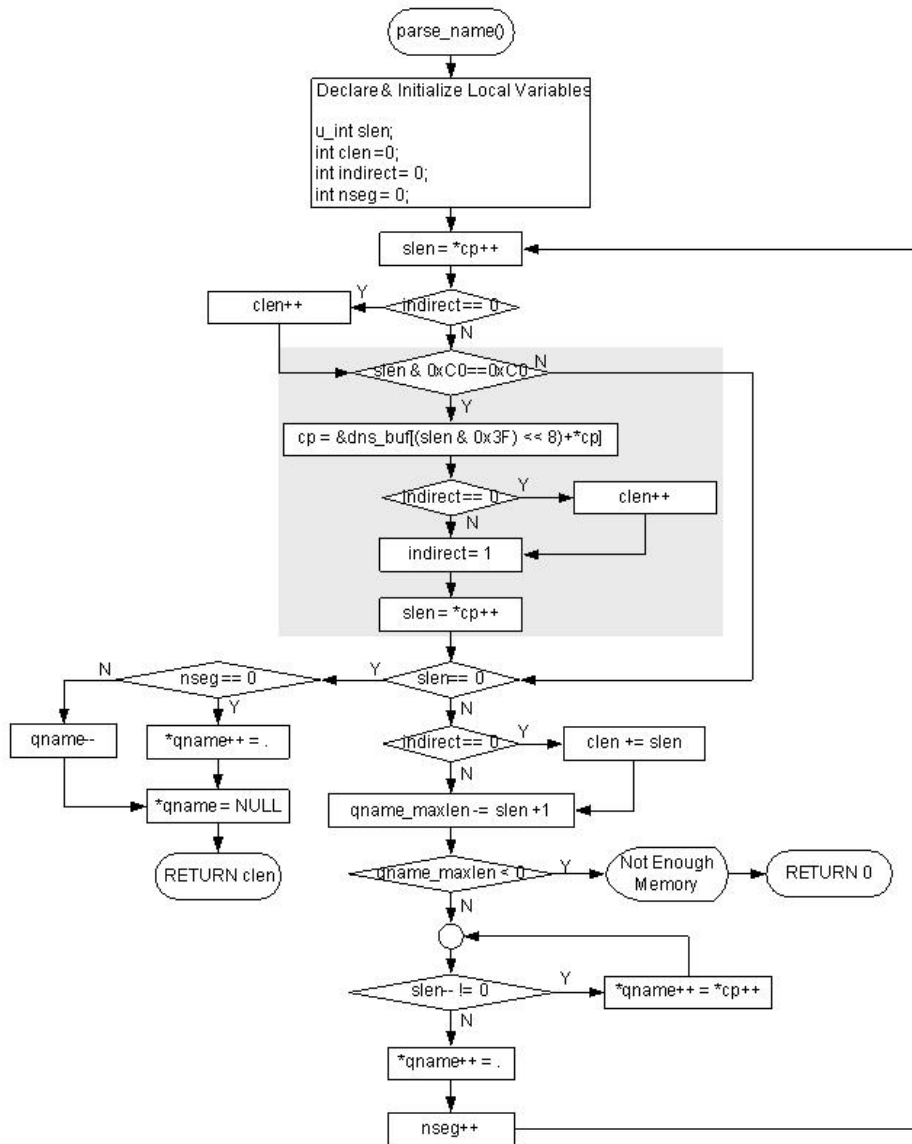
<Fig 3.44: parse_name()>
