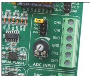
Figure 13-1: ADC module
