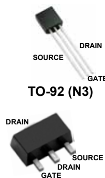
TO-243AA (SOT-89) (N8)
