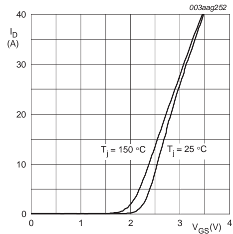
V_{DS} = 10V
