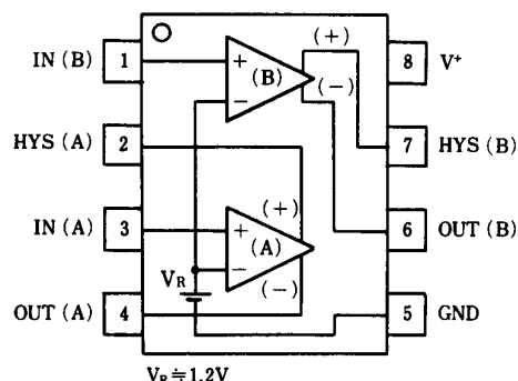
NJM2078D NJM2078M
