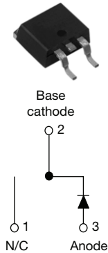
D 2 PAK
