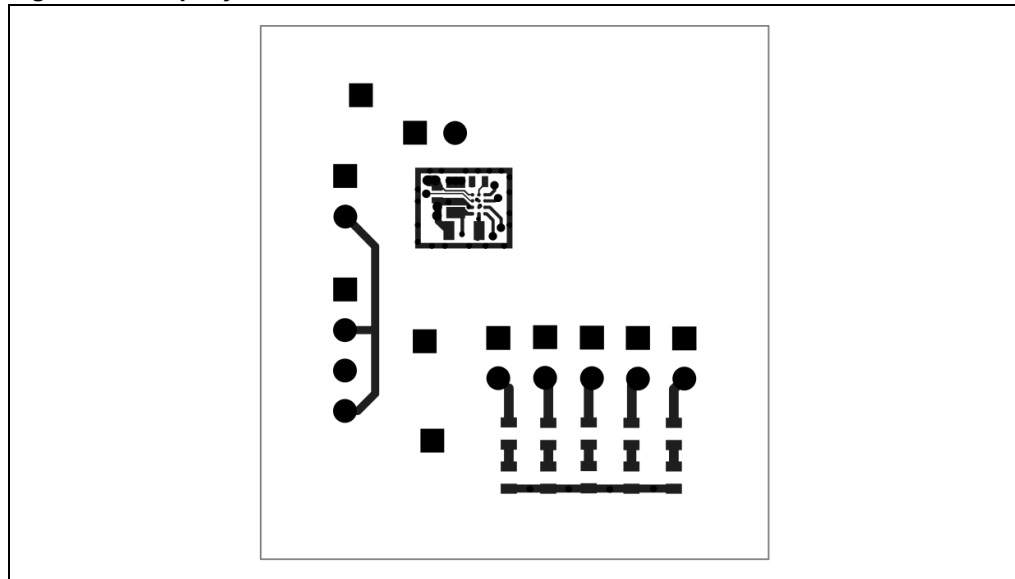
Figure 20. Top layer
